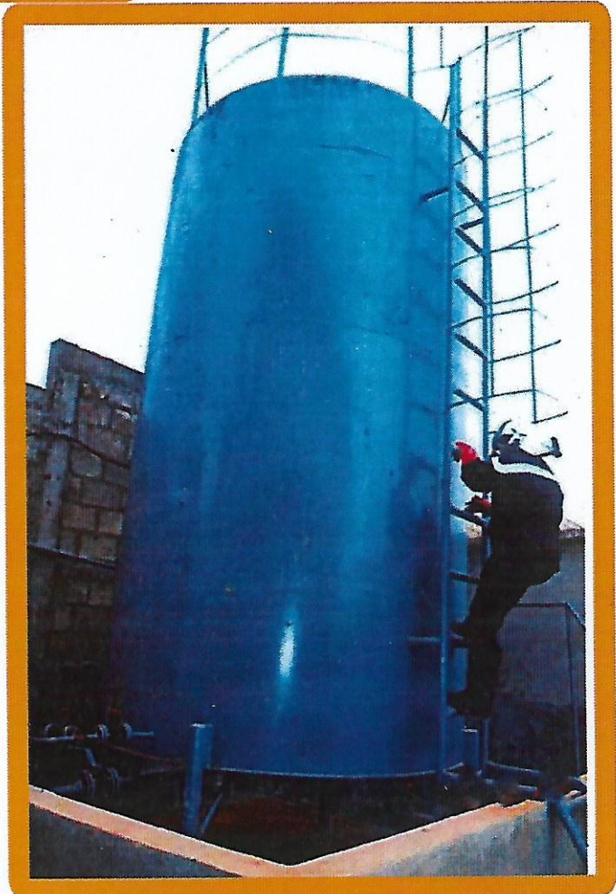
Bac de stockage déchets liquides d'une capacité de 20m3 sous rétention
